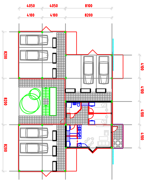
PLAN 1. ETG - 1 LEIL. TYPE B - 9 PPL.
