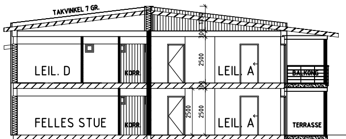
SNITT C-C 2-SIDIG LEIL./ FELLESROM
