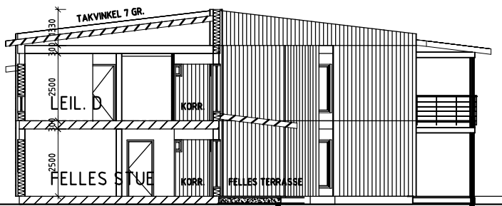
SNITT A-A VED FELLES TERRASSE
