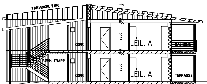
SNITT B-B GJENNOM UTVENDIG RØMN. TRAPP
