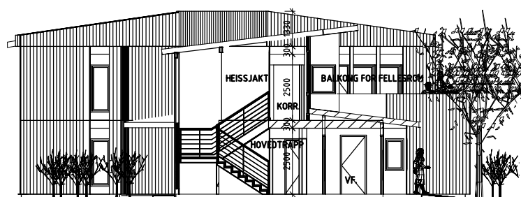
SNITT D-D GJENNOM HOVEDINNGANG / HOVEDTRAPP
