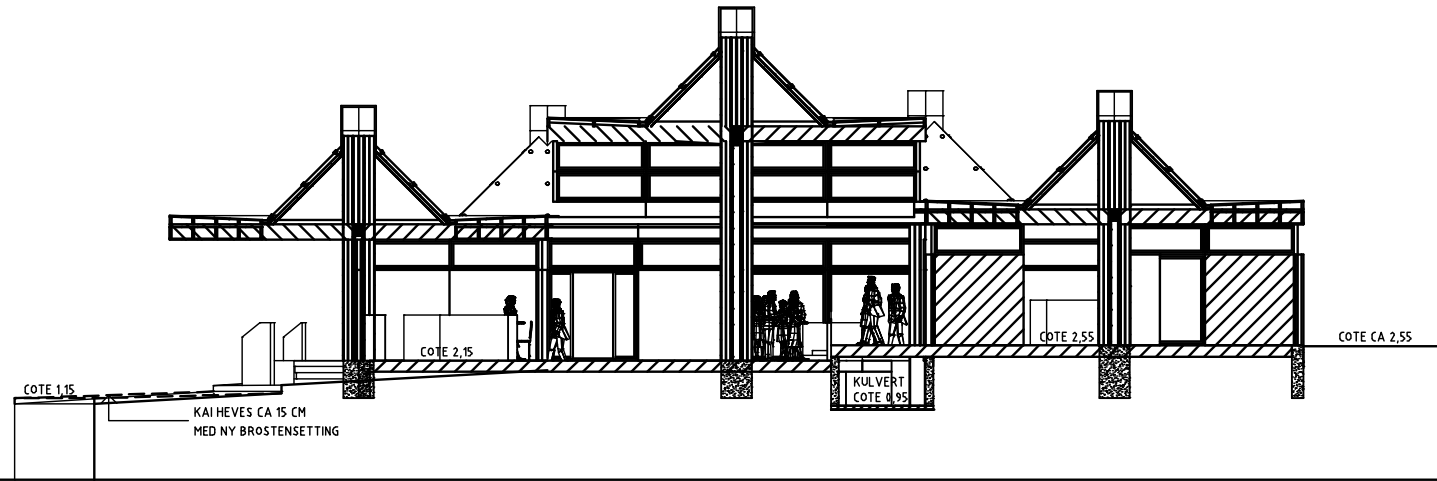
SNITT A-A
