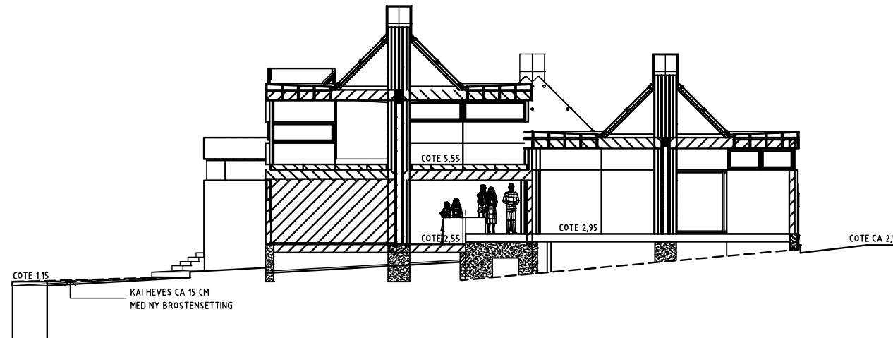
SNITT B-B
